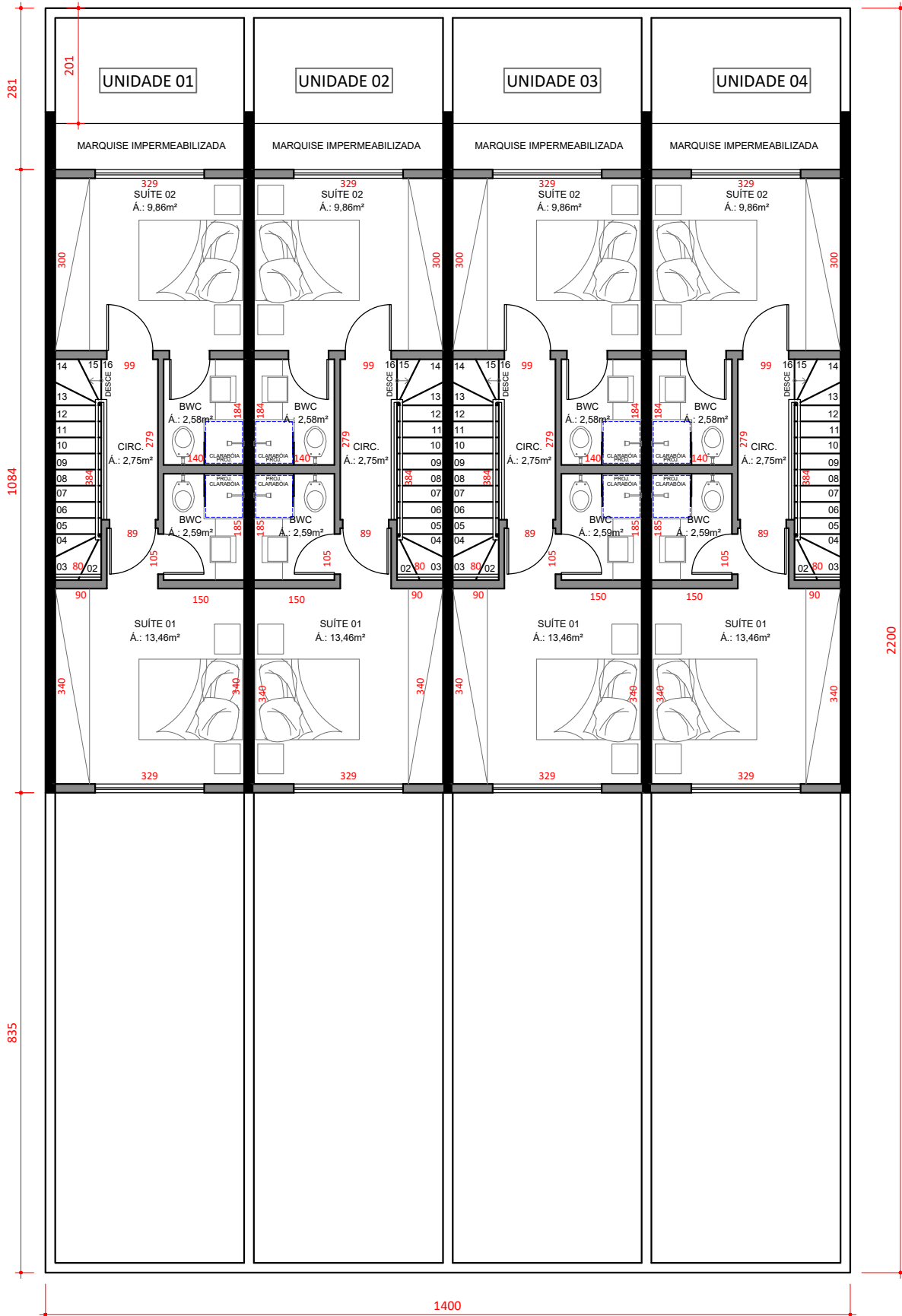
PLANTA BAIXA SUPERIOR
